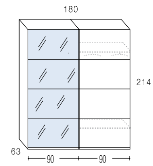
Ref. DK60L i Armario corredero 2 puertas CON LUNA IZQUIERDA
