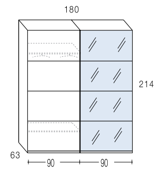
Ref. DK60L d Armario corredero 2 puertas CON LUNA DERECHA
